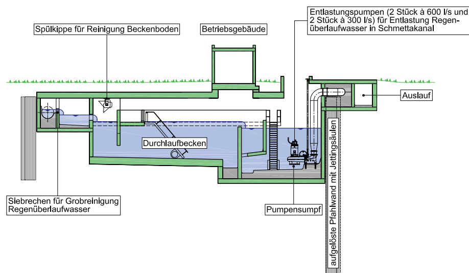
Schnitt Regenbecken mit Betriebsgebäude
